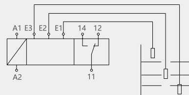
NJB1-YW 接线图
