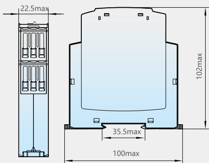
外形尺寸
