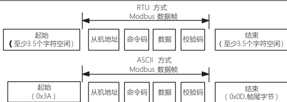
图3-4-1 Modbus协议格式
