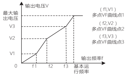
图2-5-2 自定义多点V/F曲线
