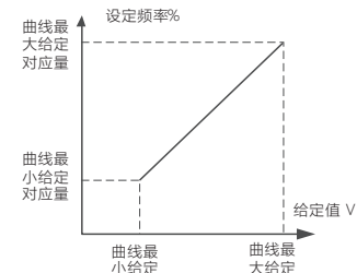
图2-2-1 AI 曲线1 设定
