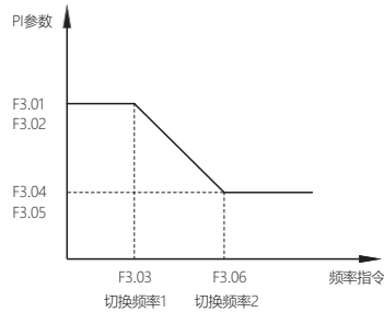
图2-6-1 速环PI参数切换示意图
