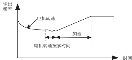
图2-3-3 转速追踪再启动时序图
