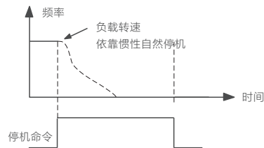
图2-3-5 自由停机时序图
