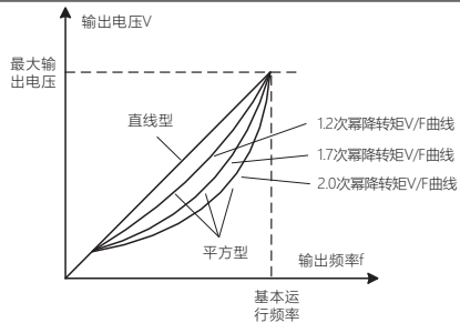
图2-5-3 降转矩V/F曲线
