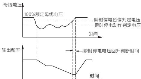
图2-12-1 瞬停不停动作示意图
