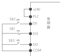
图2-1-3 三线制控制模式1
