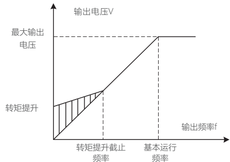
图2-5-1 通用恒转矩直线V/F曲线
