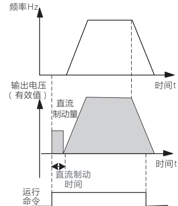
图2-3-2 先制动再启动时序图
