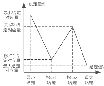
图2-2-2 AI曲线4设定
