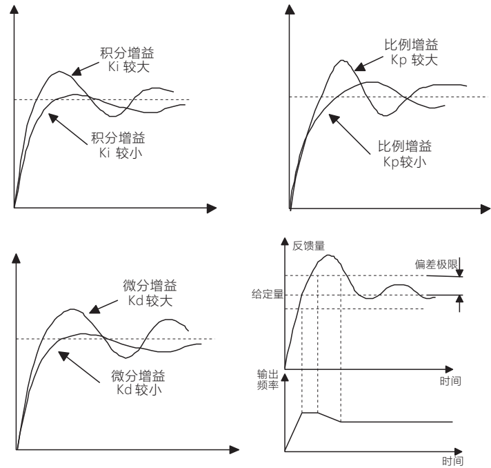
图2-2-8 过程PID参数影响示意
