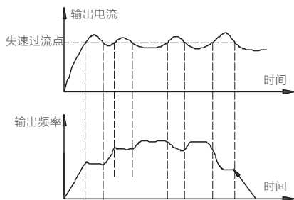
图2-7-1 过流失速动作示意图
