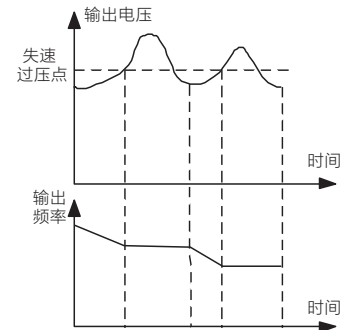
图2-8-1 过压失速动作示意图
