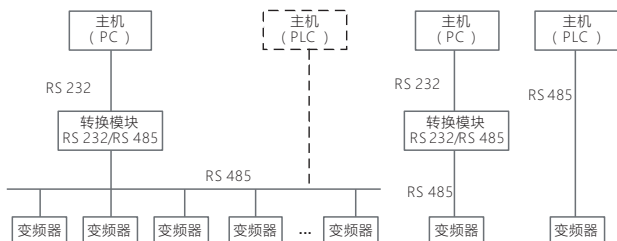
图3-1-1变频器组网方式示意图
