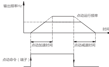
图2-13-1 点动运行示意图
