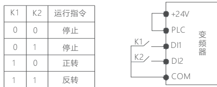
图2-1-2 两线制控制模式2
