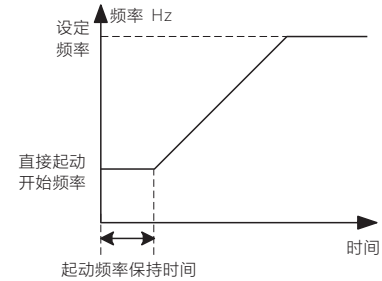
图2-3-1 直接启动时序图
