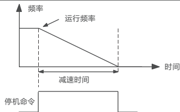
图2-3-4 减速停机时序图
