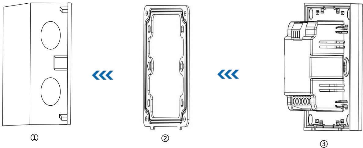
①86底盒 ②安装固定板 ③温控器本体
