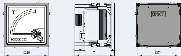
60T(C/L)666(NP80)系列外形尺寸图:
