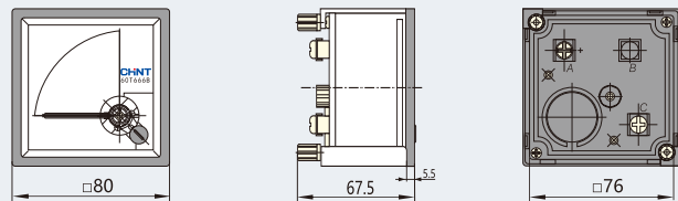
60T(C/L)666(NP80)系列外形尺寸图:
