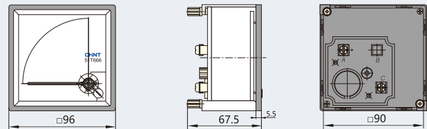
51T(C/L)666(NP96)系列外形尺寸图
