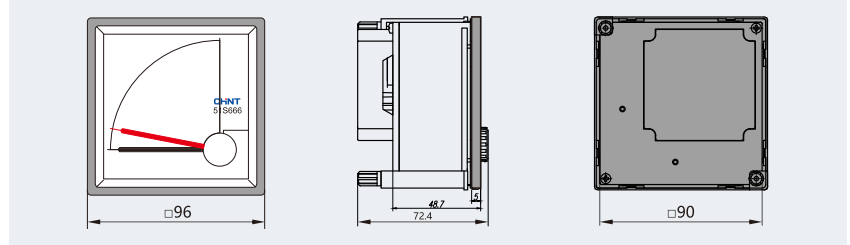
51S666外形尺寸图
