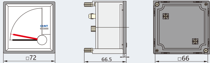
61S666外形尺寸图
